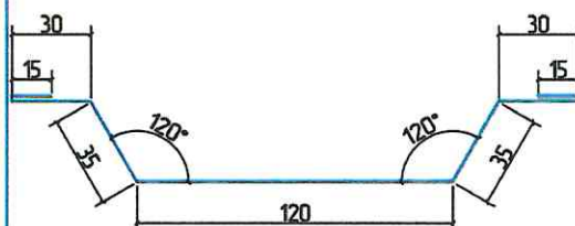
Фасонный элемент FP003
